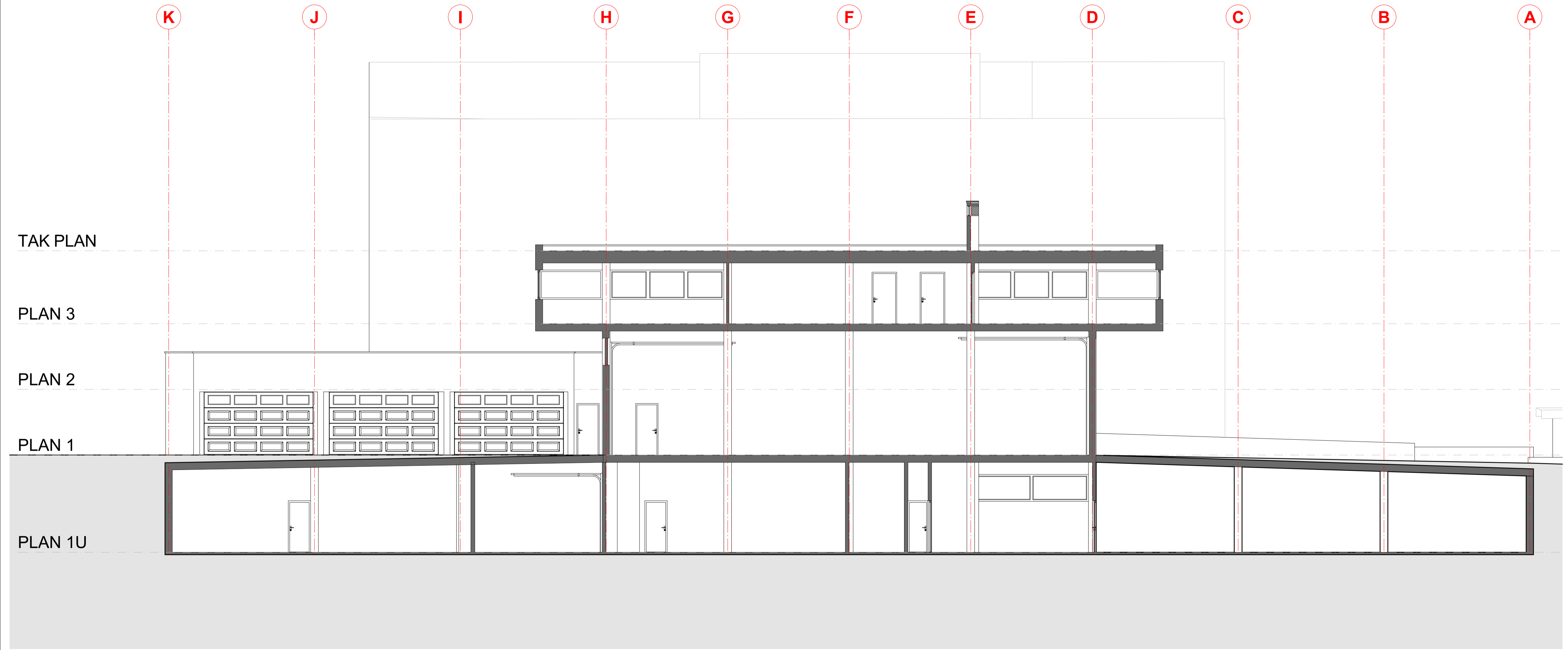
SNITT BB
