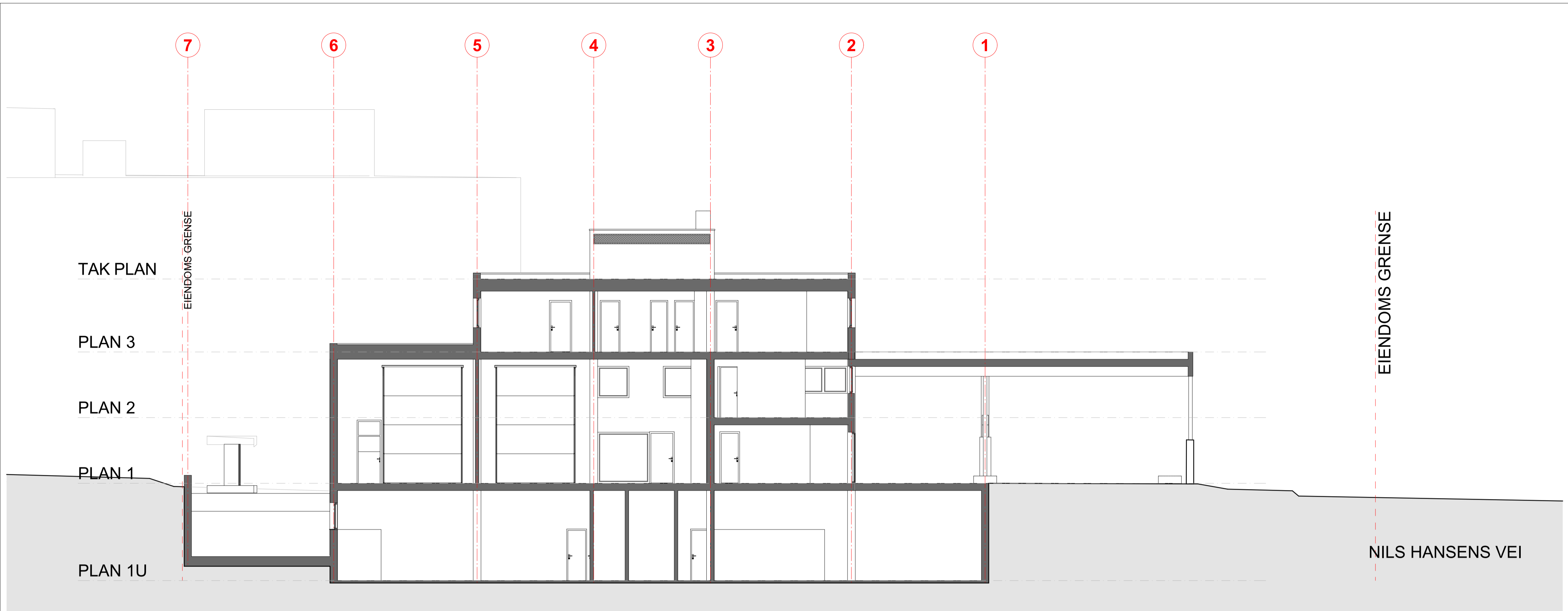
SNITT AA
